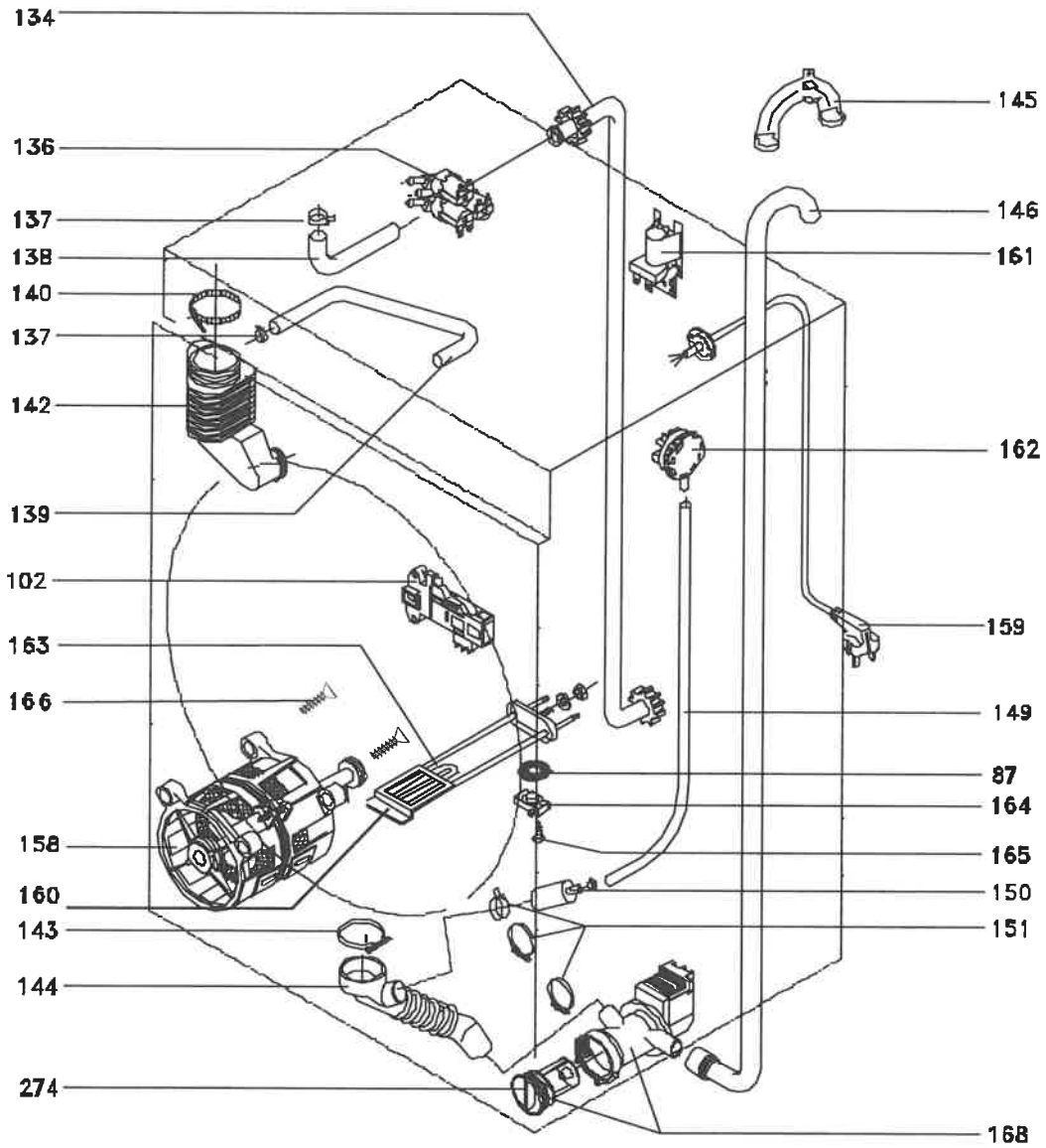
INSTALACIÓN ELÉCTRICA 322
